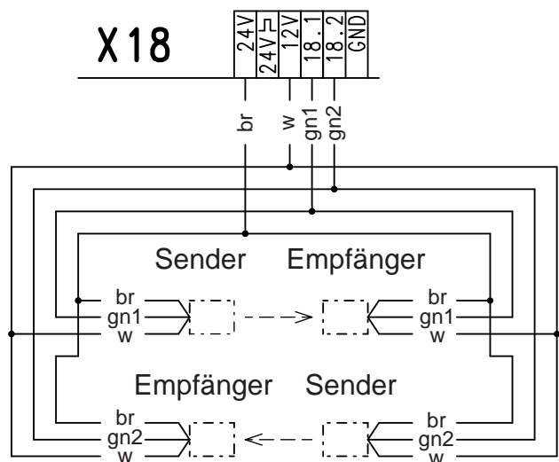
Raytor Lichtschranke oder Optische Schaltleiste als Einzugssicherung zweifach
