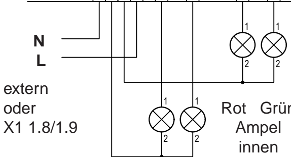
Rot Grün Ampel außen
