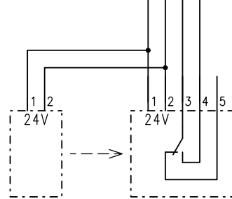
Sender Empfänger Einweglichtschranke innen oder außen
