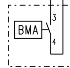
Anschluss Meldekontakt von BMA
