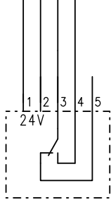
Reflexionslichtschranke innen oder außen
