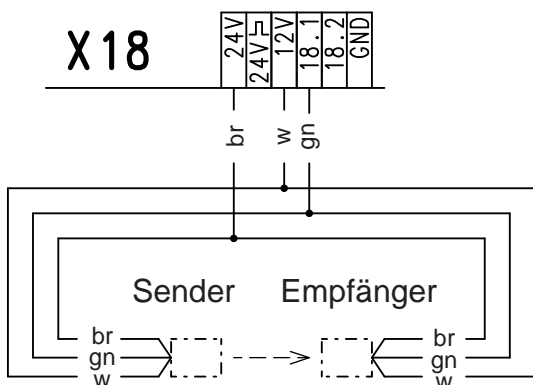
Raytor Lichtschranke oder Optische Schaltleiste als Einzugssicherung einfach
