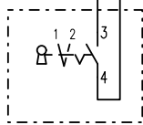
Schlüsselschalter EIN / AUS Zwischenstellung
