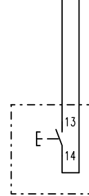
Zugschalter / Funkempfänger innen oder außen
